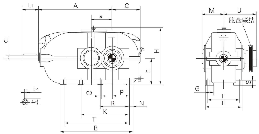
图2 DBYK型减速机（空心轴式）
