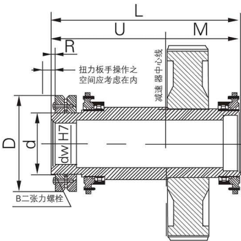
图5 DBYK、DCYK型减速机空心轴结构
