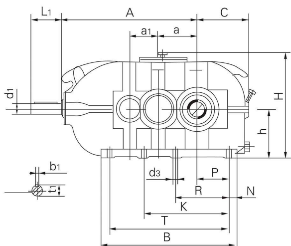
图3 DCY型减速机
