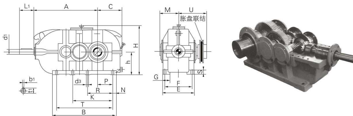
图4 DCYK型减速机（空心轴式）
