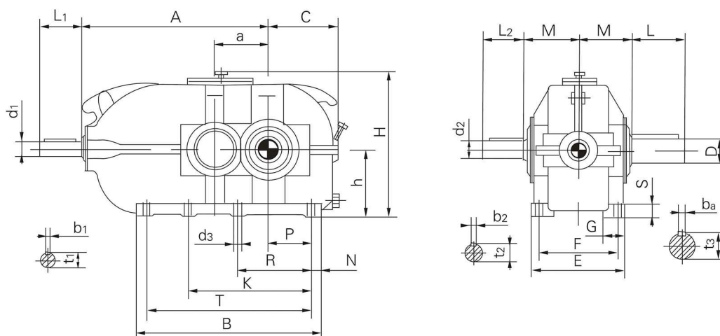
图1 DBY型减速机
