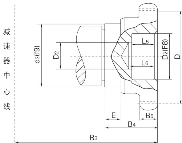
带齿轮形低速轴轴端 (C型)
